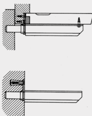
Exemples d'assemblage
