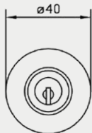
3491
