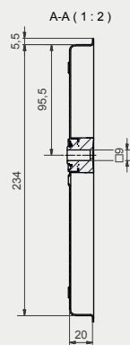
A-A (1:2)
